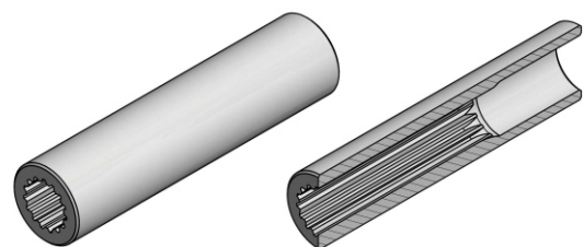
LUVA ENTALHADA
